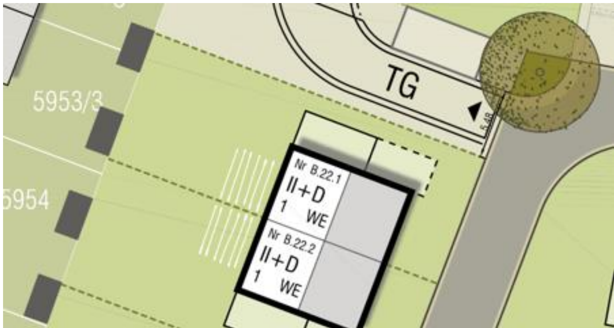
Ausschnitt aus dem Städtebaulichen Entwurf
